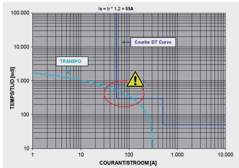
Inschakel stroompiek van een transformator.
